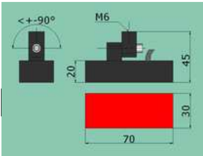
Jellemző méretek
