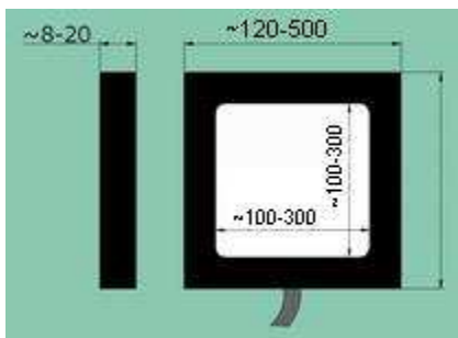
Jellemző méretek
