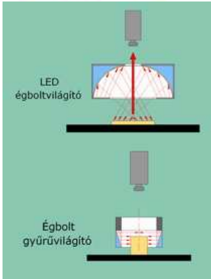
Működési példák
