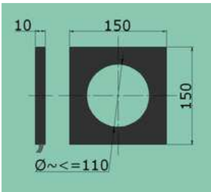
Jellemző méretek
