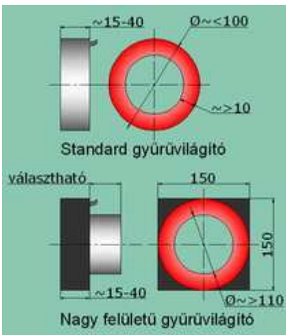
Jellemző méretek
